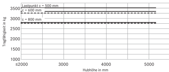
RX 60-35L Teleskop/NiHo-Hubgerüst
